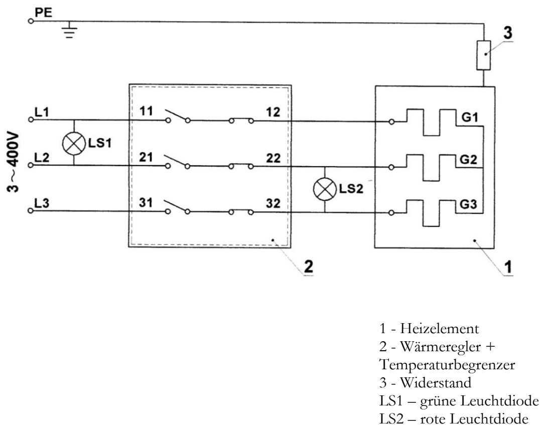
Abb. 2 Das elektrische Schema
