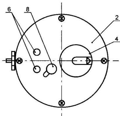
Abb.1 Aufbau der Heizpatrone.
