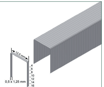
Abmessungen Type D
