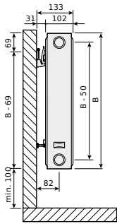
Compact Typen 20 und 22, Seitenansicht
