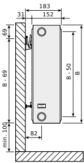
Compact Typen 30 und 33, Seitenansicht
