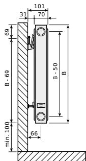
Compact Typ 21S, Seitenansicht
