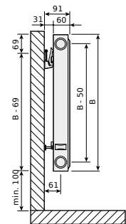
Compact Typ 11, Seitenansicht
