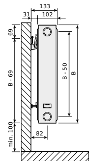
Compact Typen 20 und 22, Seitenansicht
