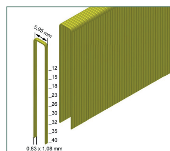
Abmessungen Type ES
