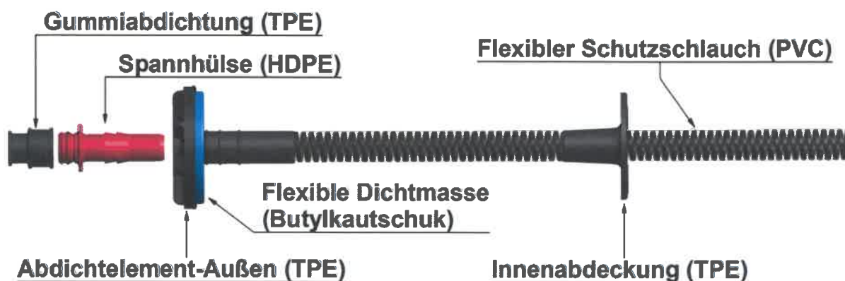
Abbildung 1: SPE-Einführung Typ SPE 16/3x7/700 (Quelle: Auftraggeber)
