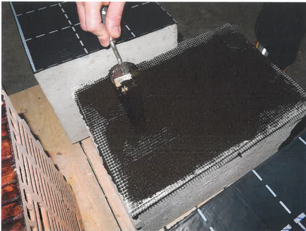
Bild 3 Einbetten der Sopro KDA 662 KellerDichtArmierung in die ersten Lage Sopro KD 752 KellerDicht 1-K
